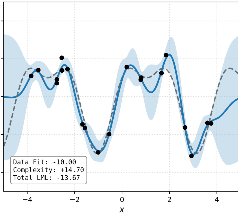
Kasus B: Optimal (Terekstrimkan oleh LML) ( l = 0.46, \sigma_n = 0.14 )
